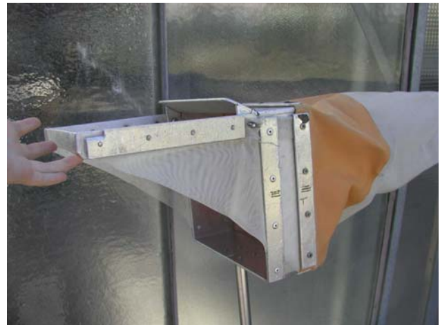
Fig. 6b. Dettaglio relativo all'intelaiatura quadrata aggiunta al retino per la raccolta quantitativa del benthos (Foto APPA BZ).
