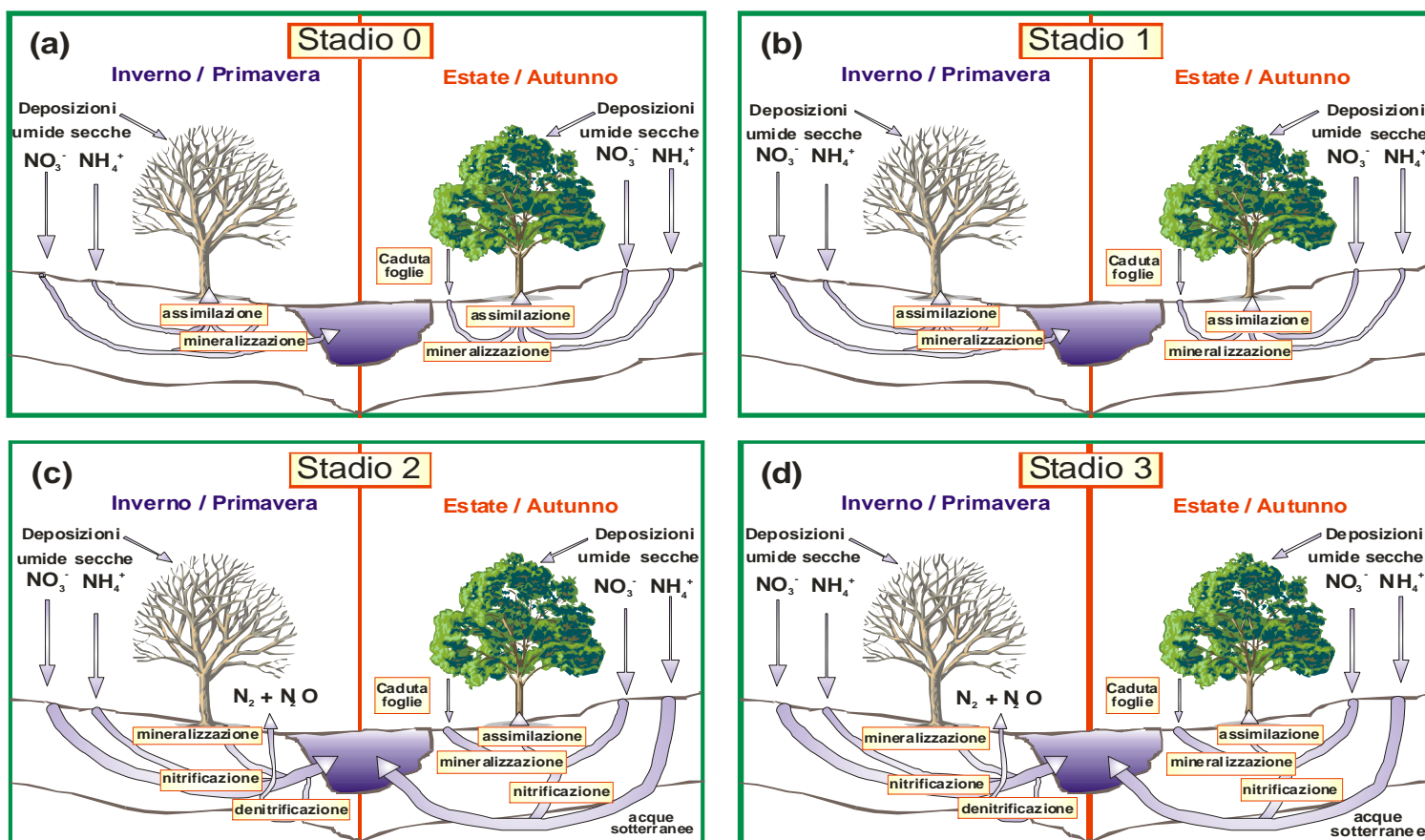
Fig.5 Rappresentazione schematica del ciclo dell'azoto di un bacino idrografico, suddiviso in quattro stadi di saturazione: (a) Stadio 0; (b) Stadio 1; (c) Stadio 2 e (d) Stadio 3 (tratto da Traaen & Stoddard, 1995).
